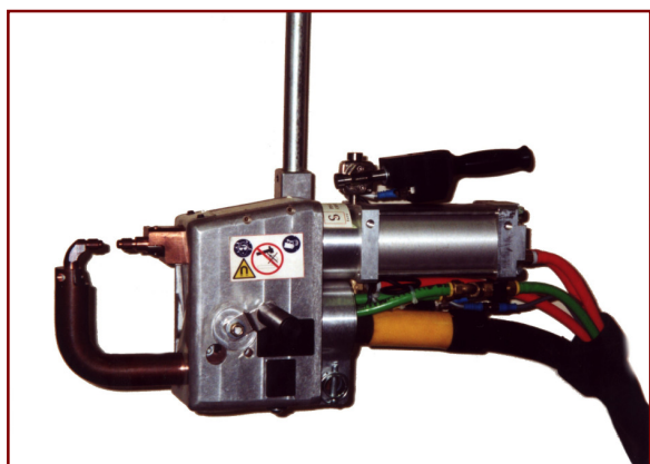
Pince en Cé C-type gun C-zange
